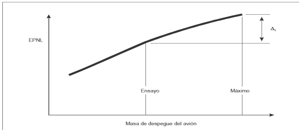
Figura A1-10. Corrección de la masa de despegue correspondiente al EPNL.-
