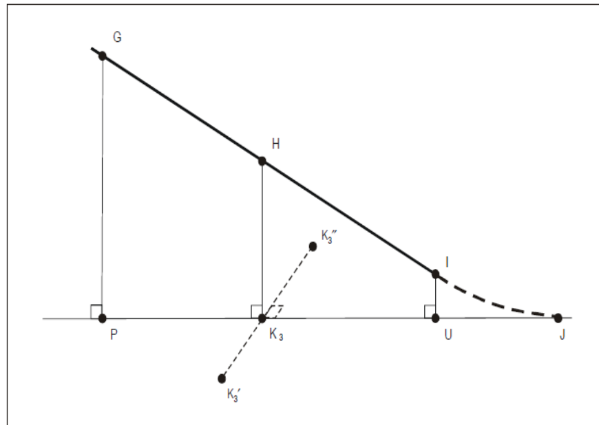
Figura A2-9. Características del perfil de aproximación de referencia para helicópteros.-
