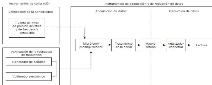
Figura C-1. Sistema de medición del ruido.-
