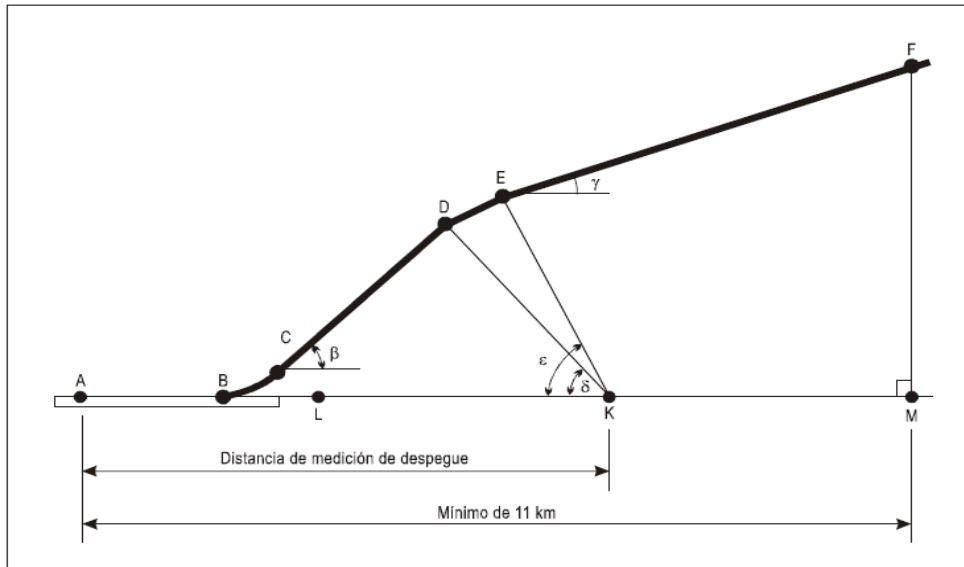
Figura A1-4. Perfil de despegue medido.-
