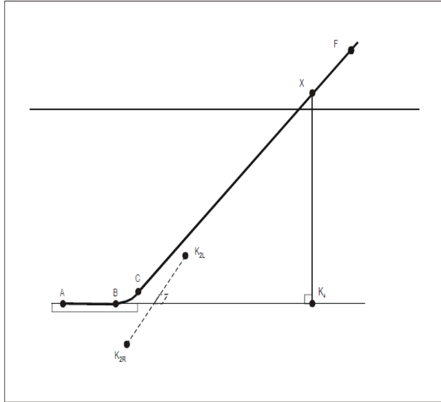
Figura A2-4. Características del perfil de ruido lateral con plena potencia de referencia para aviones.-
