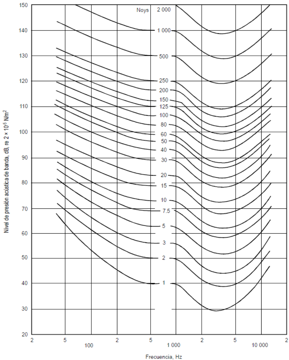
Figura A5-1. Curvas de ruido percibido.-
