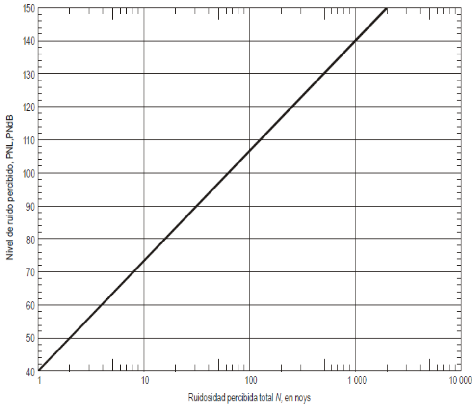
Figura A1-1. Nivel de ruido percibido en función de la ruidosidad percibida total.-
