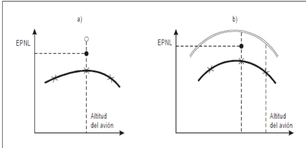
Figura A2-13. Corrección de asimetría lateral.-
