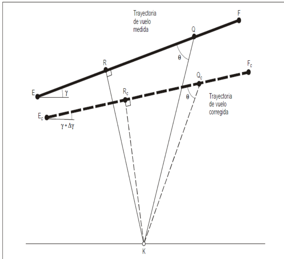
Figura A1-6. Características del perfil de despegue que influyen en el nivel acústico.-
