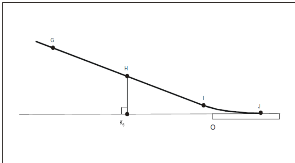
Figura A2 -6. Características del perfil de aproximación de referencia para aviones.-
