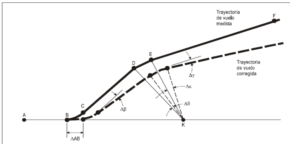
Figura A1-5. Comparación de los perfiles de despegue medidos y corregidos.-
