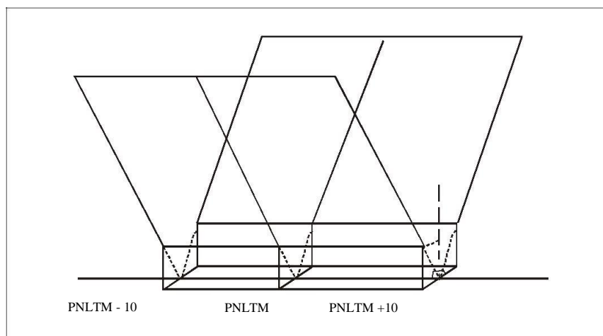
Figura 8-1. Tolerancias de desviación lateral de helicópteros.-
