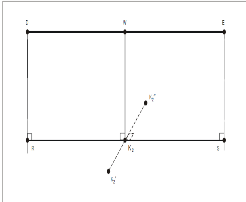
Figura A2-8. Características del perfil de sobrevuelo de referencia para helicópteros.-
