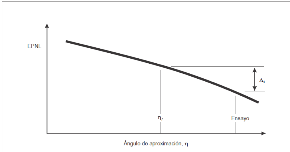
Figura A1 – 12. Corrección del ángulo de aproximación correspondiente al EPNL.-
