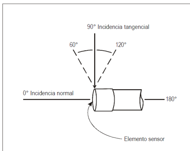
Figura A2-1. Ilustración de los ángulos de incidencia sonora en un micrófono.-
