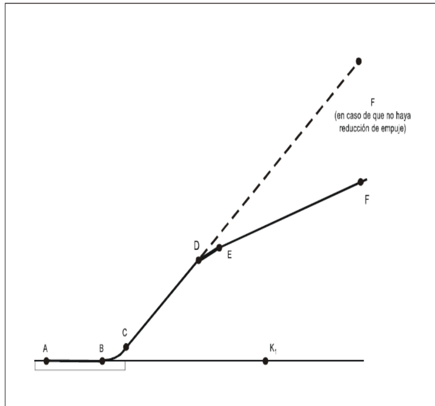
Figura A2-5. Características del perfil de sobrevuelo de referencia para aviones.-
