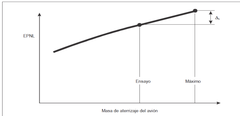
Figura A1-11. Corrección de la masa de aproximación correspondiente al EPNL.-
