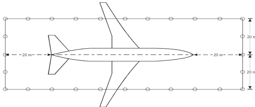
Figura C-2. Rectángulo de puntos de medición del ruido.-
