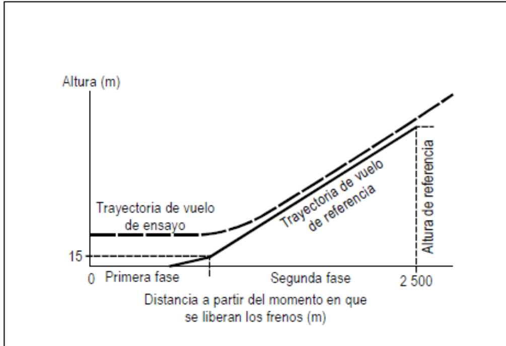
Figura A6-1. Perfiles de ensayo y de referencia típicos.-
