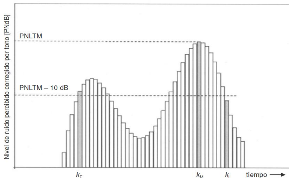
Figura A2-2. Ejemplo de historial de tiempo de ruido en sobrevuelo.-
