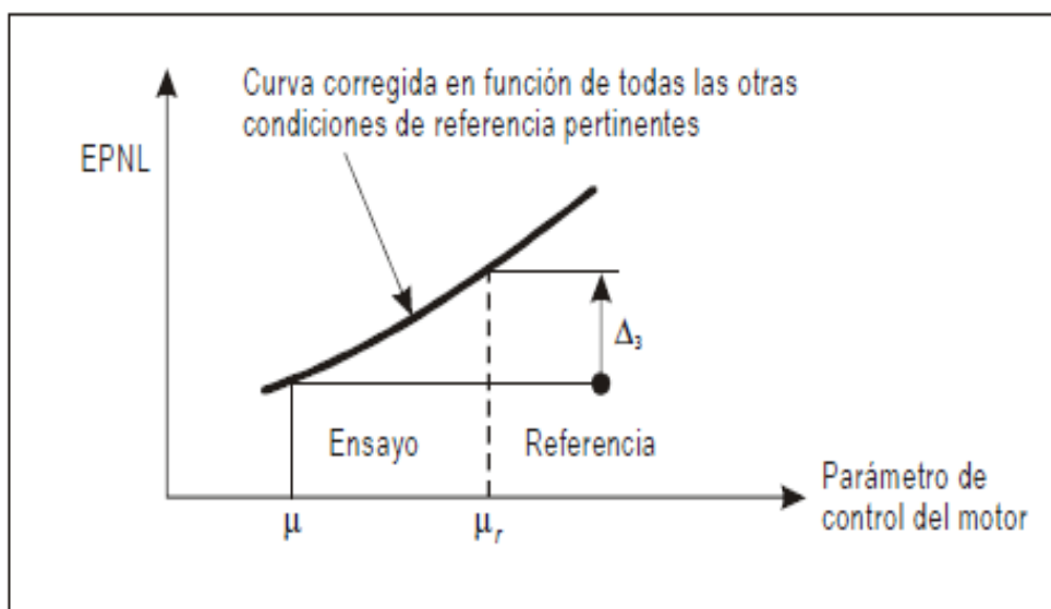
Figura A2-12. Ajuste del ruido en la fuente.-
