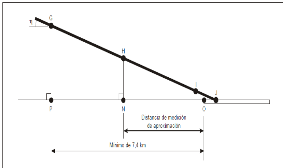
Figura A1 -7. Perfil de aproximación medido.-
