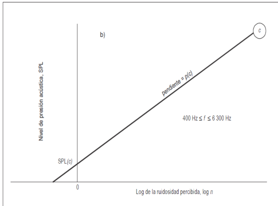
Figura A1-3. Nivel de presión acústica en función de la ruidosidad percibida.-
