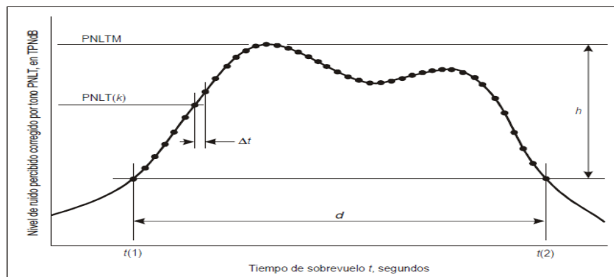
Figura A1-2. Ejemplo del nivel de ruido percibido corregido por tono en función del tiempo de sobrevuelo de la aeronave.-
